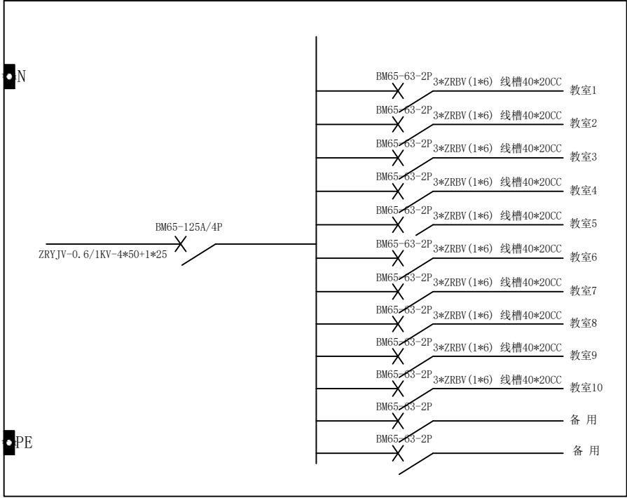
教学楼1~5层配电箱系统图
