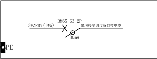
教学楼空调配电箱系统图
