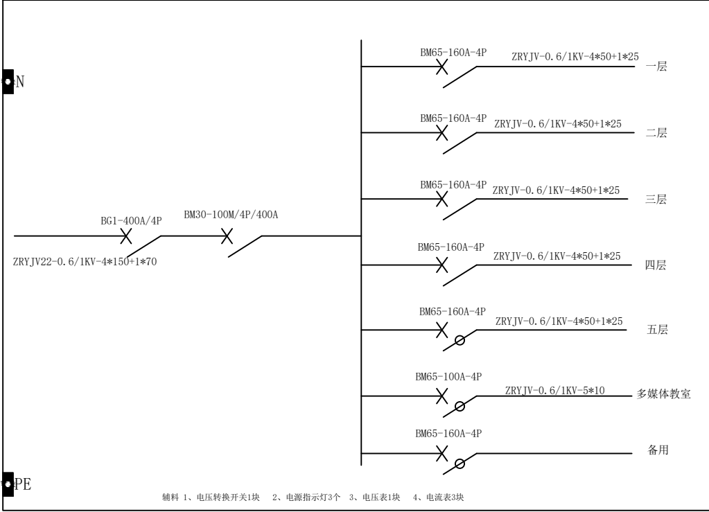
教学楼总配电箱系统图
